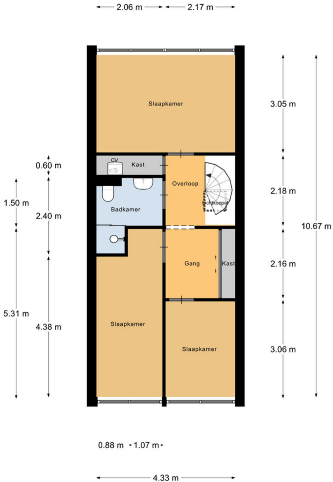
Tweede Verdieping
